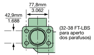
Vista C-C
